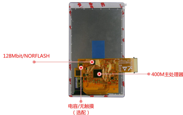
图 1-3 硬件配置图
