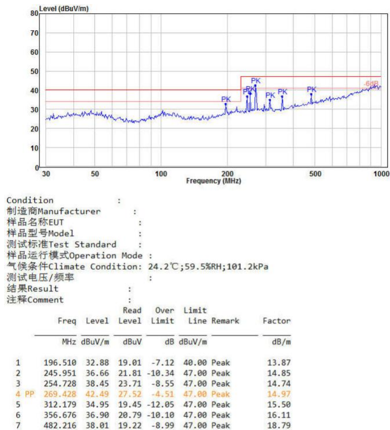
图 6-5 RE 测试水平方向
