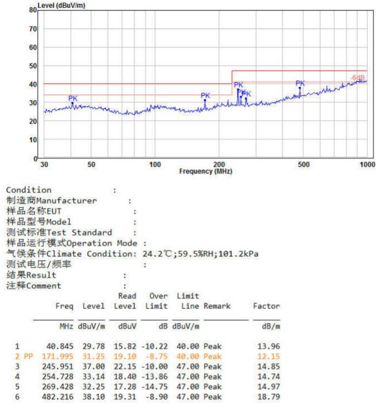
图 6-6 RE 测试垂直方向
